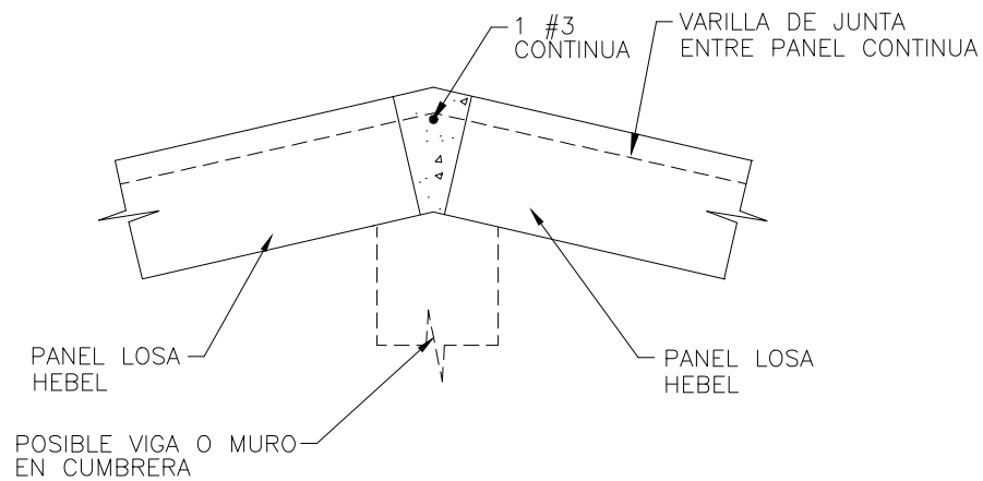
ELEVACION
