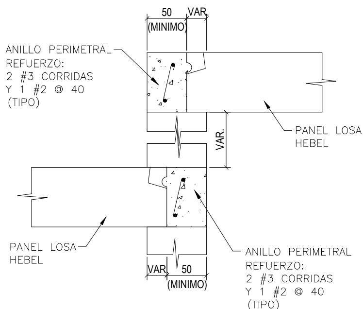
ELEVACION
