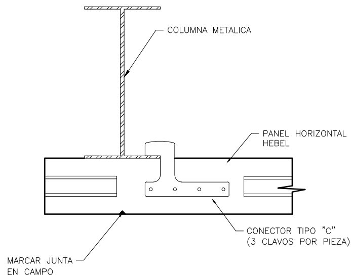
PLANTA
