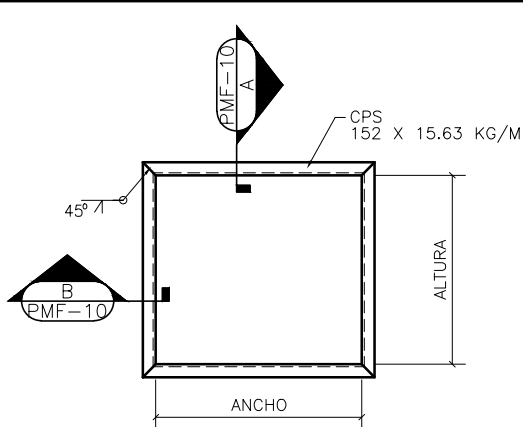
DETALLE DE HUECO
