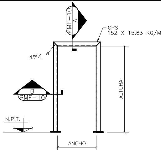
DETALLE DE PUERTA
