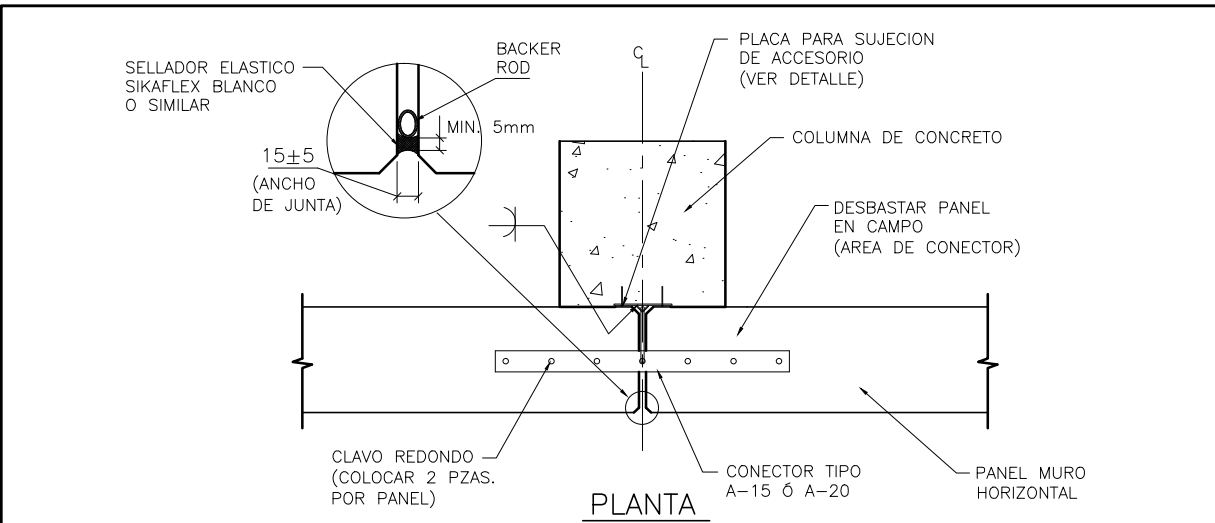
PLANTA CONEXION DE PANEL DE MURO S/E
