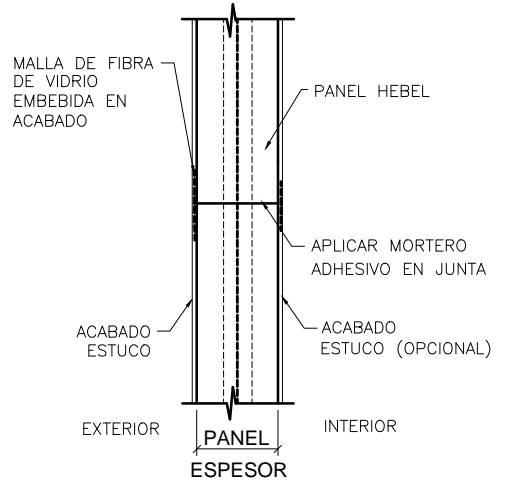
JUNTA ENTRE PANELES S/E
