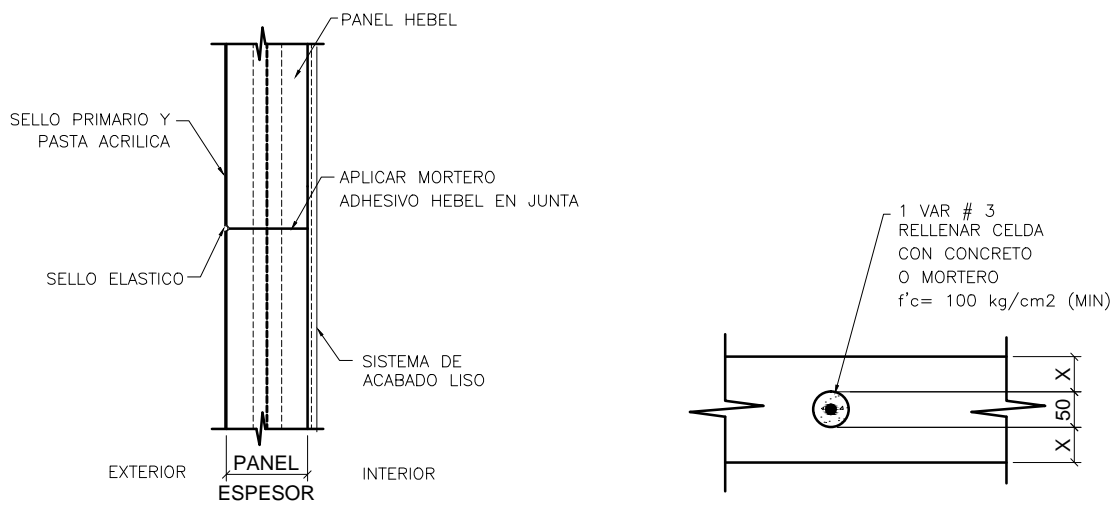
B JUNTA ENTRE PANELES PMF-13B S/E
