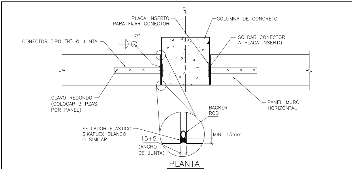
PLANTA CONEXION DE PANEL DE MURO A COLUMNAS PMF-13B S/E
