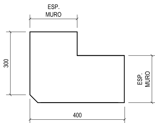
DIMENSIONES
