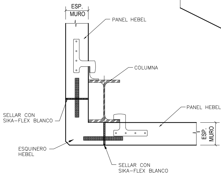
PLANTA
