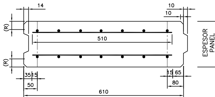
CORTE TRANSVERSAL
