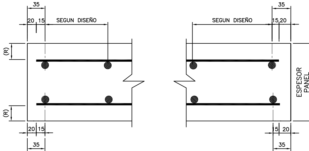
CORTE LONGITUDINAL
