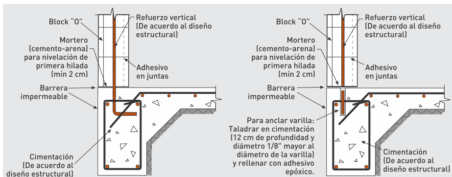
Fig. 7: Anclaje de refuerzo vertical en cimentación.
