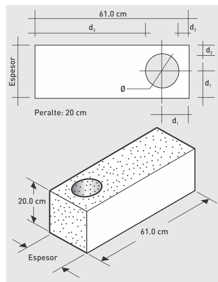
Fig. 2: Block "O" Hebel para refuerzo vertical.
