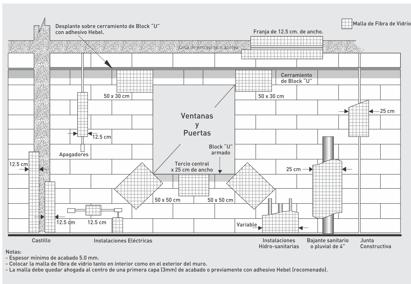
Fig. 27: Ubicación típica de la malla de fibra de vidrio en Mampostería Reforzada Hebel.
