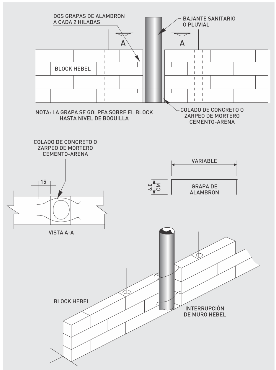
Fig. 23: Detalle de bajante sanitario o pluvial.
