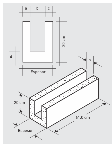
Fig. 3: Block "U" Hebel para refuerzo horizontal.
