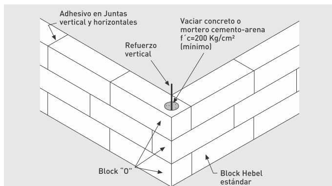
Fig. 8: Refuerzo vertical en esquinas.
