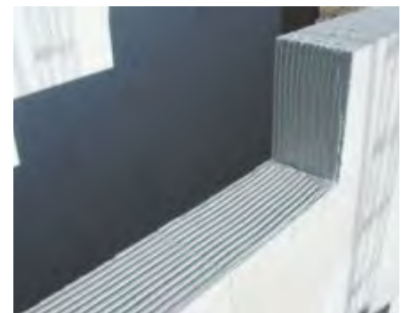
Fig. 8: Adhesivo aplicado en cara horizontal y vertical (a todo lo largo y ancho del block).
