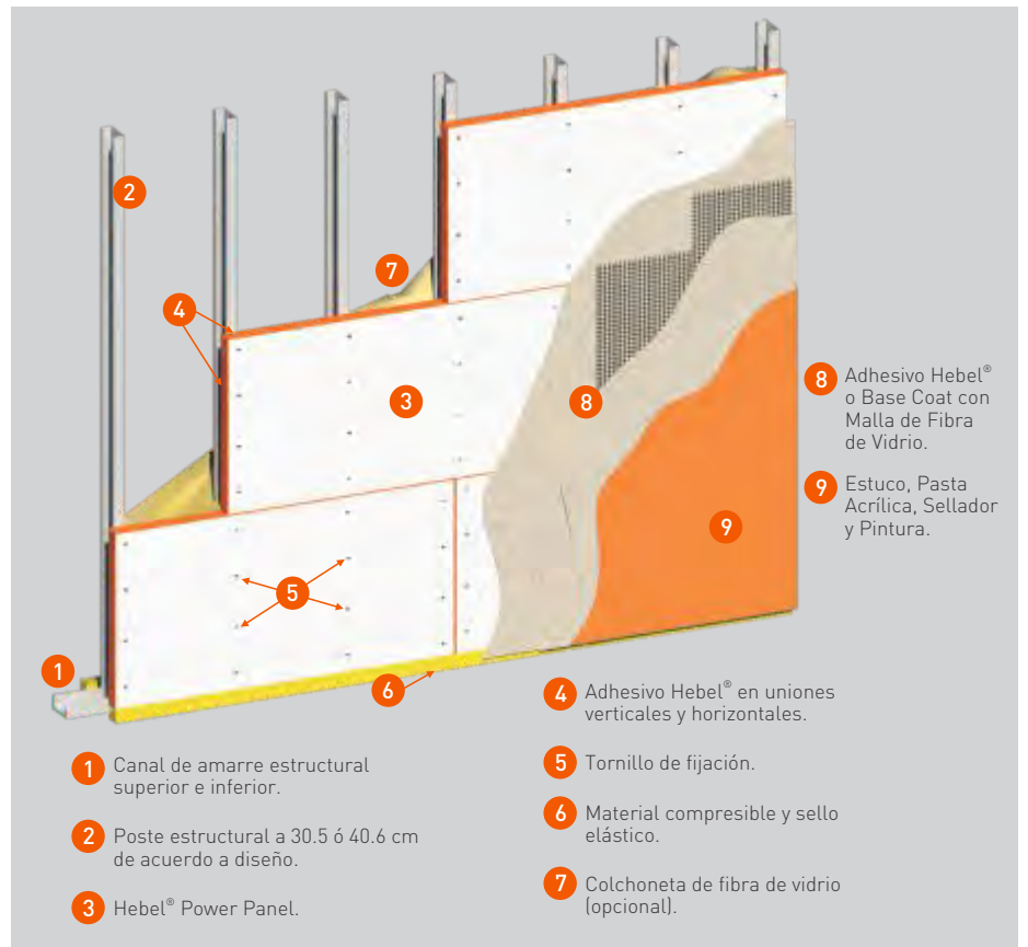
Fig. 22 Muro Exterior
