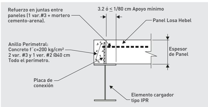
Fig. 18: Detalle de anillo perimetral en elemento de acero.
